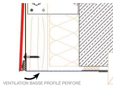
DÉTAIL LINTEAU
