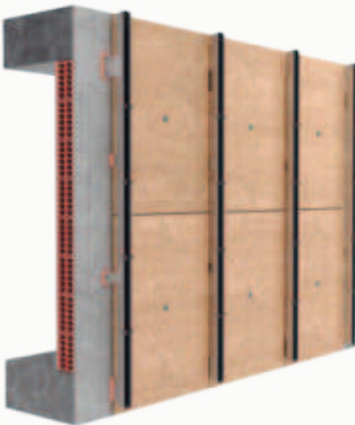
Instalación de los perfiles verticales. Installation of vertical profiles. Installation des profils verticaux. Установка вертикальных профилей.
