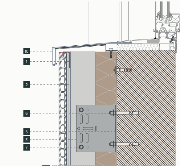
C sección vertical. vertical section. section verticale. вертикальный разрез
