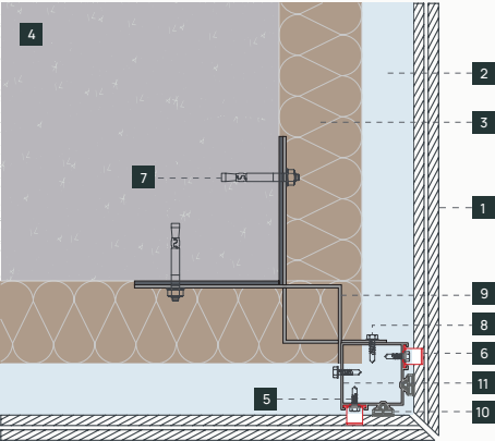
sección horizontal. horizontal section. section horizontale. горизонтальный разрез.
