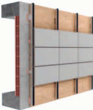
Colocación de las piezas cerámicas. Fitting the ceramic panels . Placement des pièces en céramique. Установка керамических плит.
