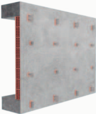
Replanteo y colocación de las ménsulas. Layout and fising of the brackets and insulation. Implantation et fixation des supports. Разметка и монтаж кронштейнов.
