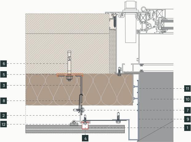
A sección horizontal. horizontal section. section horizontale. горизонтальный разрез.
