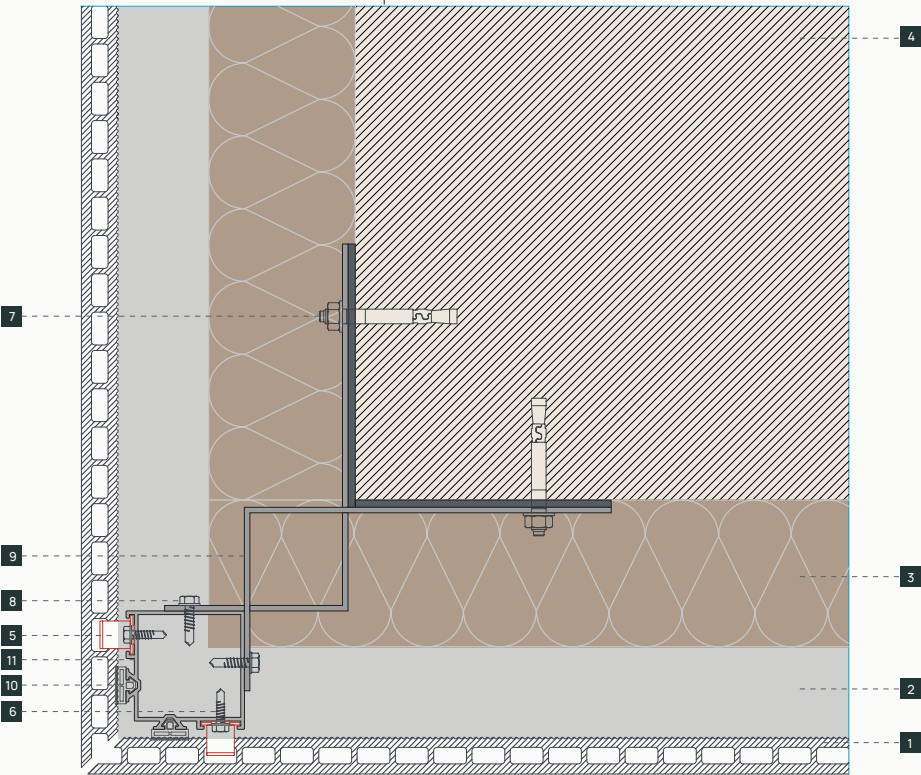
sección vertical. vertical section. section verticale. вертикальный разрез
