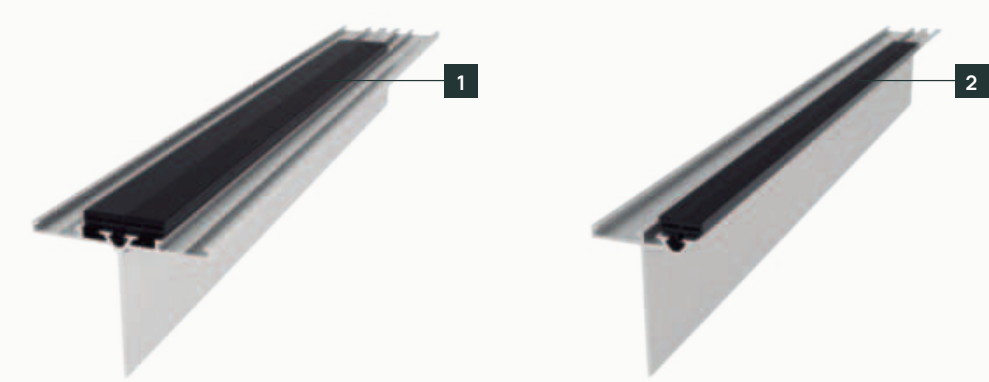
Perfil vertical "T" acanalada "T" grooved vertical profile Profil vertical rainuré en "T" Вертикальный профиль с пазом "Т"
