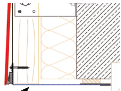
VENTILATION BASSE PROFILÉ PERFORÉ
