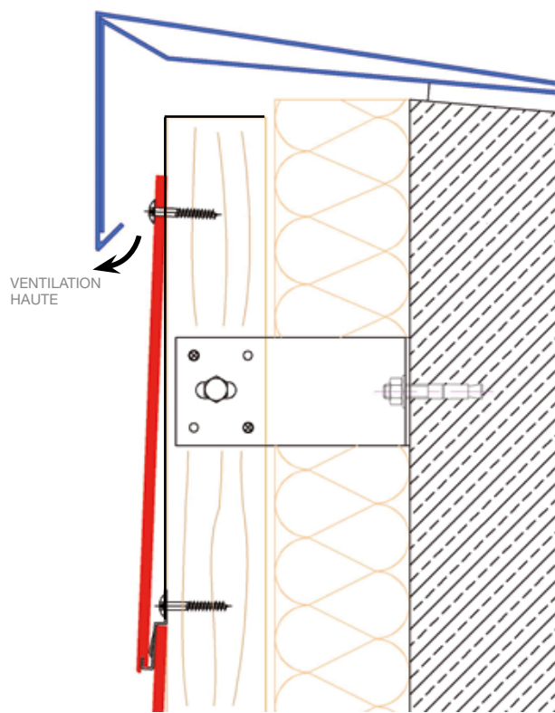
DÉTAIL COUVERTINE
