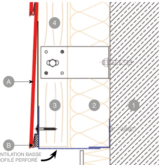
DÉTAIL DÉPART BAS
