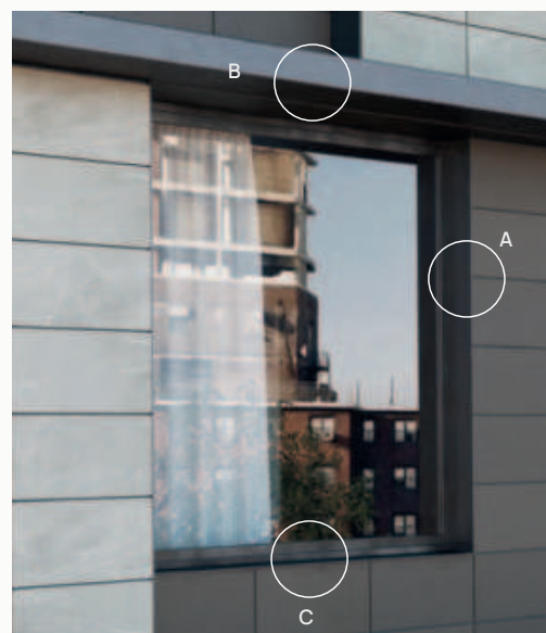
VENTANA CON VIERTTEAGUAS METÁLICO. WINDOW WITH METALLIC SILL. FENÊTRE AVEC APPUI MÉTALLIQUE. ОКНО С МЕТАЛЛИЧЕСКИМ РАЗЛИВОМ.
