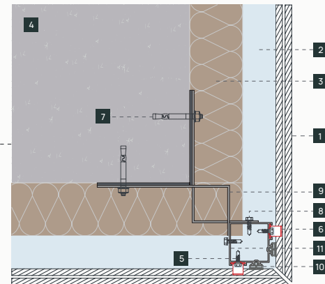
sección horizontal. horizontal section. section horizontale. горизонтальный разрез.
