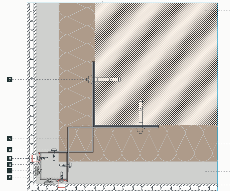
sección vertical. vertical section. section verticale. вертикальный разрез.
