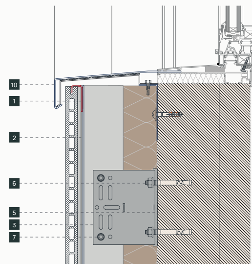
C sección vertical. vertical section. section verticale. вертикальный разрез
