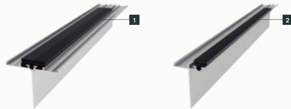
Perfil vertical "T" acanalada "T" grooved vertical profile Profil vertical rainuré en "T" Вертикальный профиль с пазом "Т"
