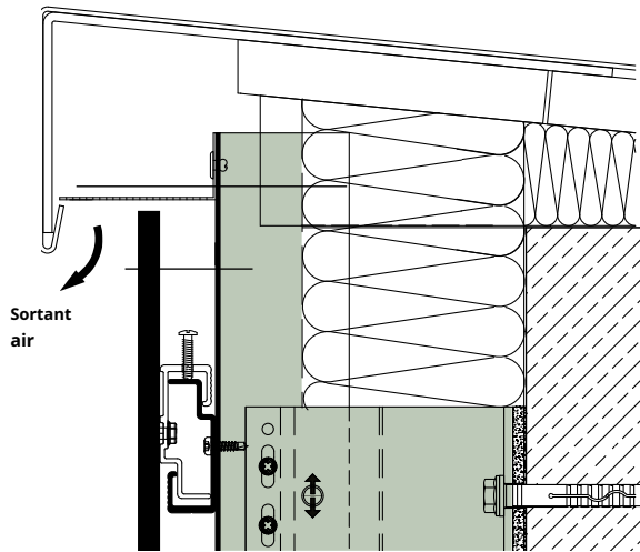
Fascia A109
